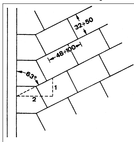
FIG. 26 - Sistemazione di un lastricato a giunti inclinati
